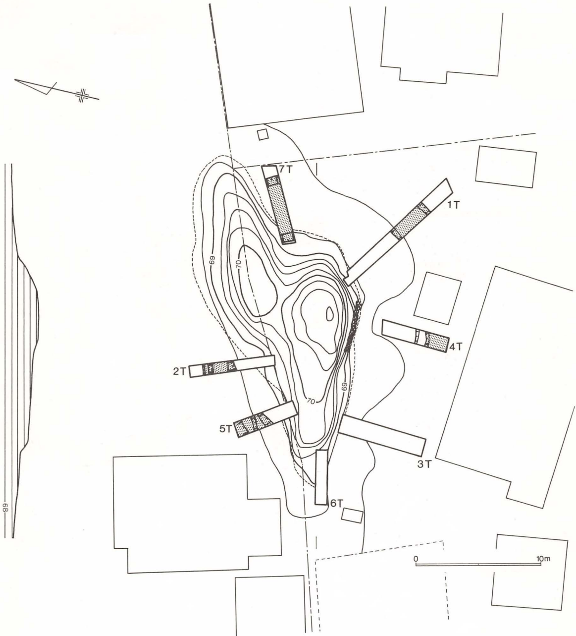
第2図 川本町箱崎4号墳測量図
