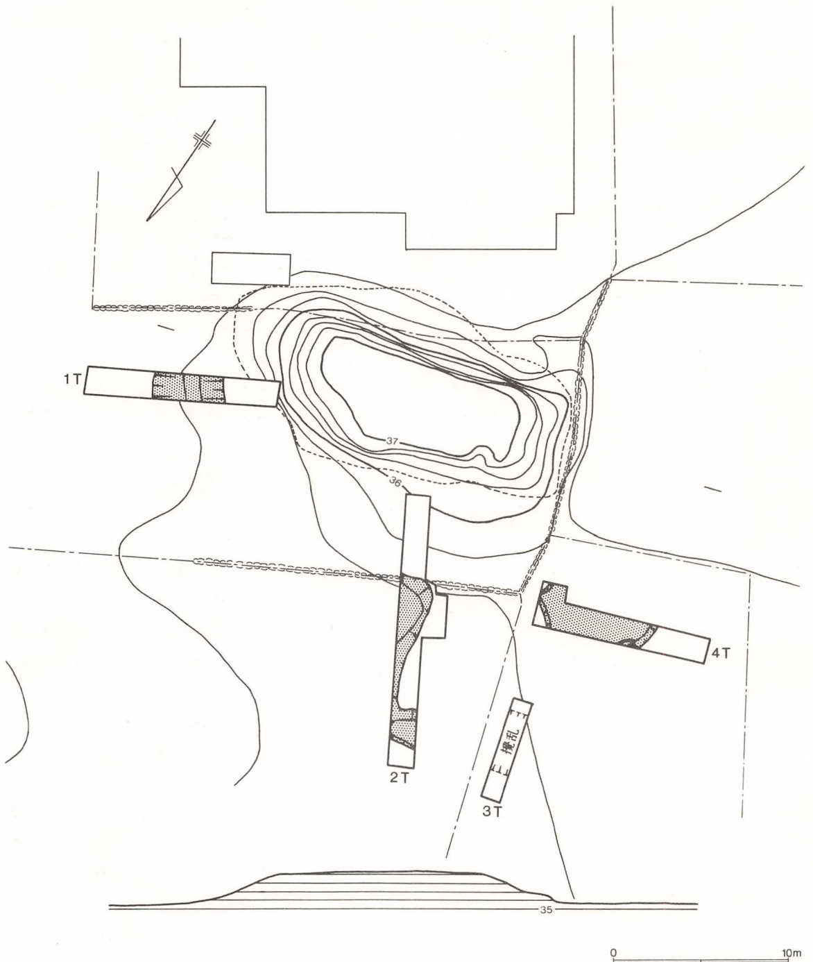
第3図 深谷市木の本10号墳測量図
