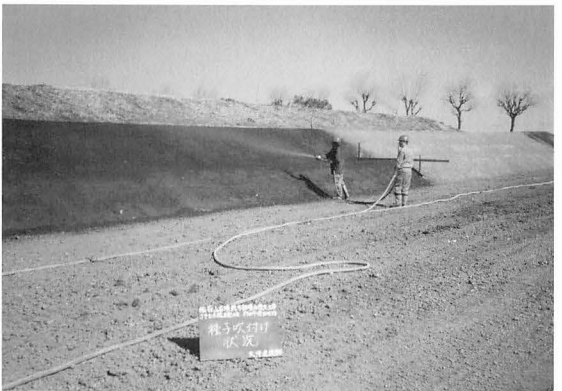
12年度 種子吹付け工事
